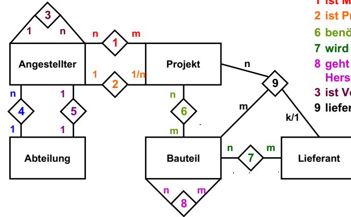
Beispiel 7.7: „ER-Diagramm“ (Ausschnitt aus einem Unternehmen)
