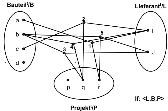
Dreier-Beziehung aus Beispiel 7.3: (Verallgemeinerung auf Grad > 2)
